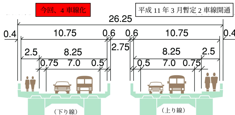
断面図
